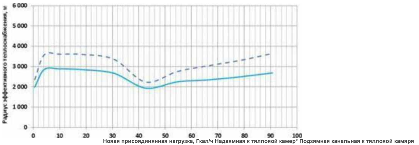
Рисунок 5.3 - Влияния способа прокладки на эффективный радиус
