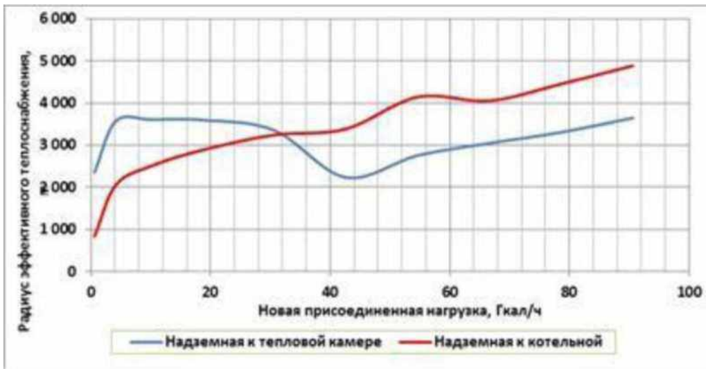
Рисунок 5.2 - Зависимость эффективного радиуса от присоединенной нагрузки
